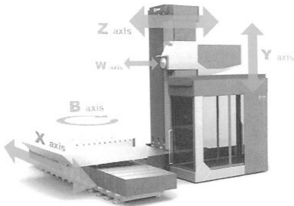
Abbildung 2: Technische Parameter der Maschine – Vorschube
